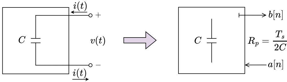
Εικόνα 2.4: Αναπαράσταση WDF πυκνωτή
