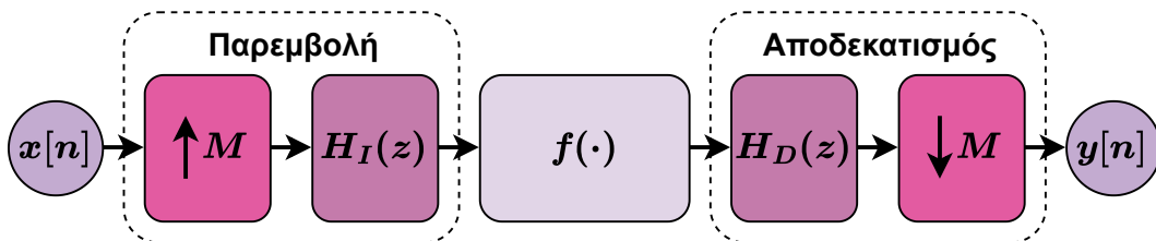
Εικόνα 2.17: Διαδικασία υπερδειγματοληψίας
